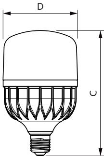
Bulb 120-240V 50-W 4500lm 6500K E27 ND
